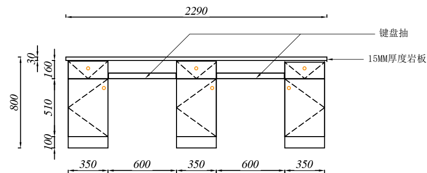
小圆弧柜立面图
