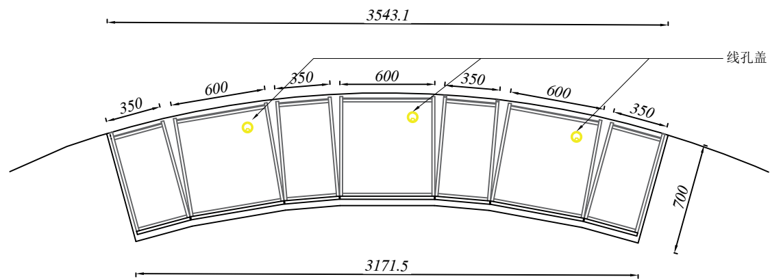
大圆弧柜平面图
