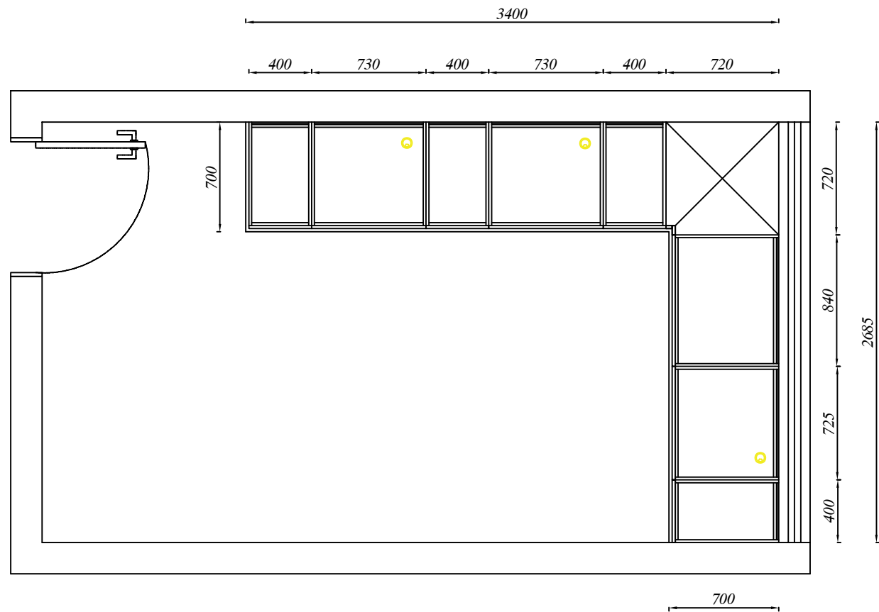
南①平面图
