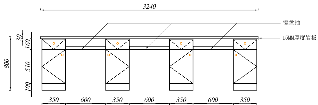
大圆弧柜立面图
