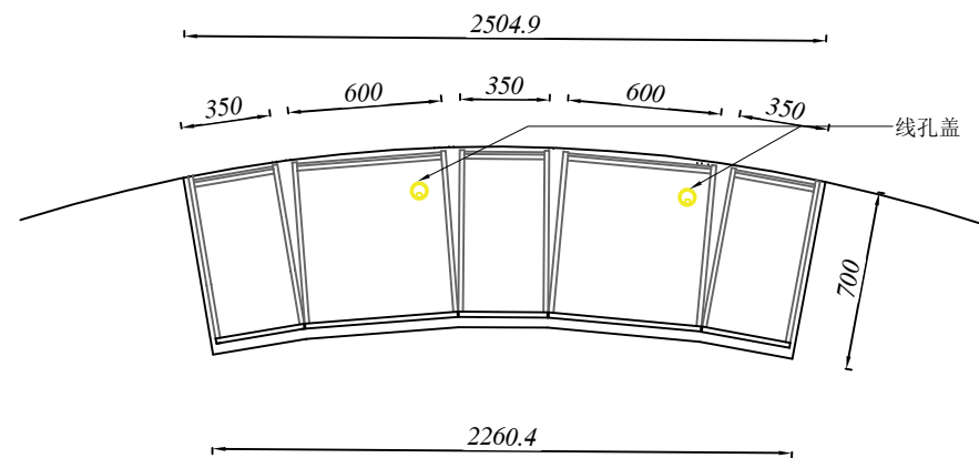
小圆弧柜平面图
