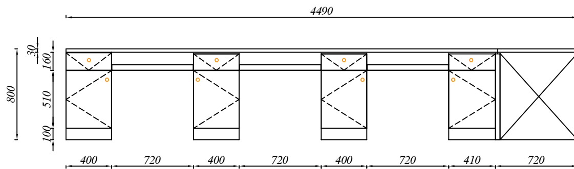
北②立面图
